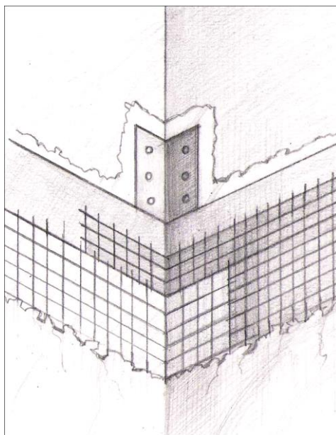
Рисунок 17 – Установка уголков
