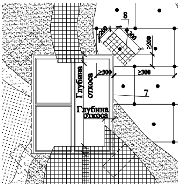
Рисунок 18 – Защита углов оконных (дверных) откосов
