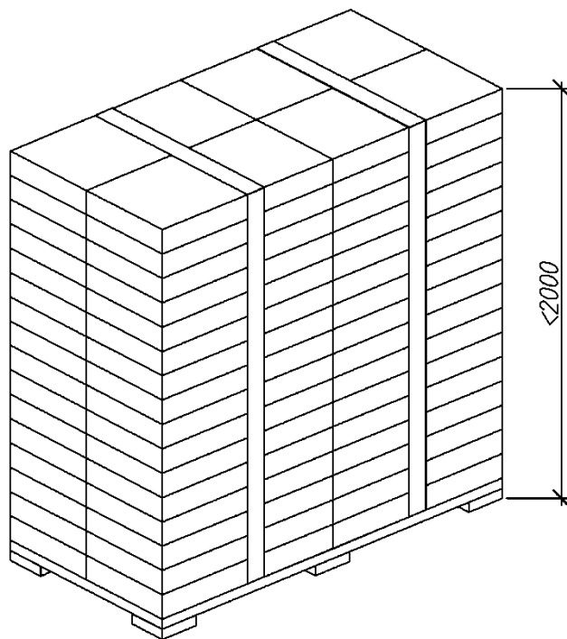
а - рулонов стеклосетки; б - плит утеплителя Рисунок 4 – Схема складирования материалов
