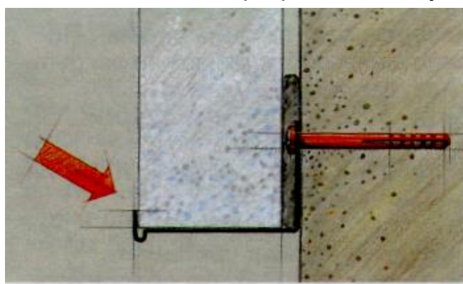
Рисунок 12 – Расположение теплоизоляционных плит нижнего ряда
